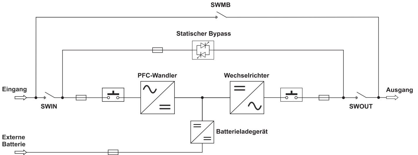
Schaltbild der USV mit einem Eingang (ohne separaten Bypass)
