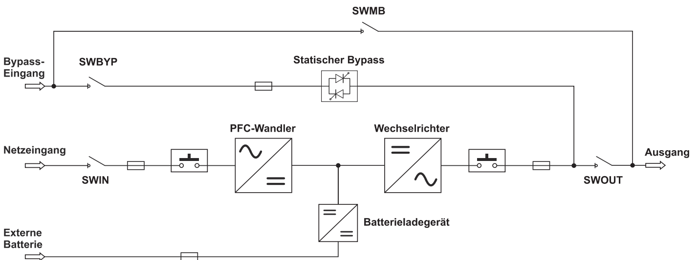
Schaltbild der USV mit zwei Eingängen (mit separatem Bypass)
