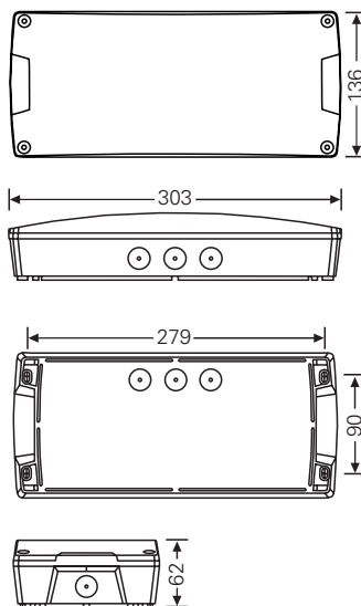
Massangaben in mm
