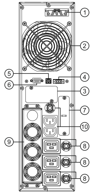
SDU 8 kVA u. 10 kVA
