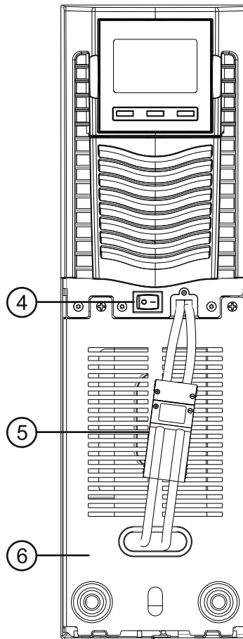
SDU 5 u. 6 kVA ohne Frontplatte
