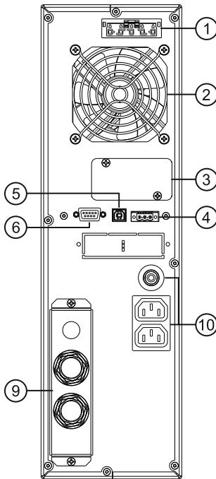
SDU 5 kVA u. 6 kVA mit Festanschluss für Ein- und Ausgang, und Energy Share Buchsen
