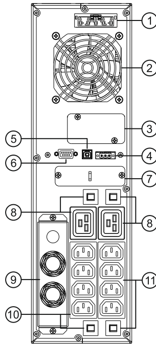
SDU 5 kVA u. 6 kVA mit Festanschluss für Ein- und Ausgang, inkl. Steckdosen und Energy Share Buchsen
