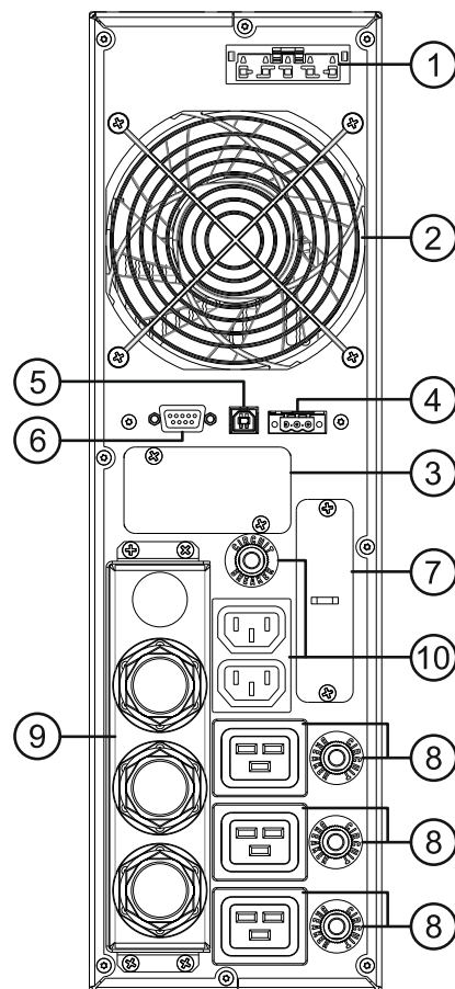
8 – 10 kVA Modell
