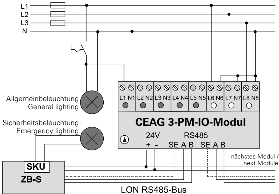
Bild 3 / fig. 3: Schaltung eines CEAG 3-PM-IO Moduls / Wiring of the CEAG 3-PM-IO module
