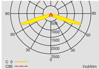
Lichtverteilungskurve SL i-P65 LED O CG-S mit symmetrischer Optik
