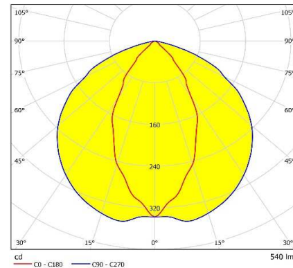
Lichtverteilung TS5-LED CGS comp./PLC
