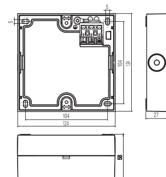
Zusatzgehäuse
