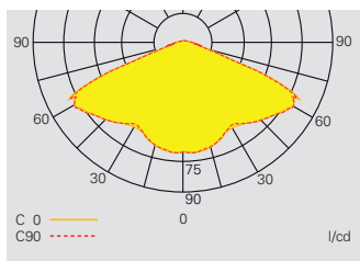
Lichtverteilungskurve GuideLed SL 13022.2 CG-S Einbau mit symmetrischer Optik
