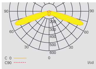
Lichtverteilungskurve GuideLed SL 13012.2 CG-S Einbau mit asymmetrischer Optik
