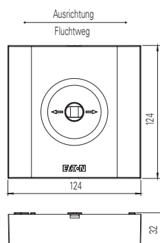
Massangaben in mm
