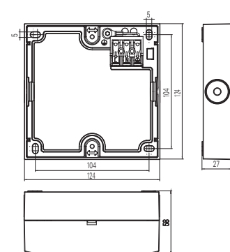
Zusatzgehäuse
