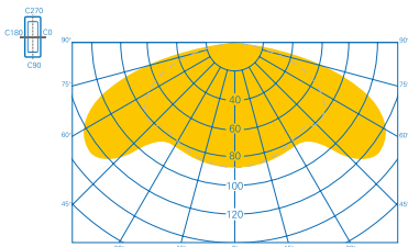
Lichtverteilungskurve
