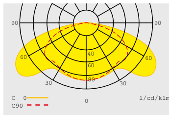
Lichtverteilungskurve FlexiTech SU CG-S
