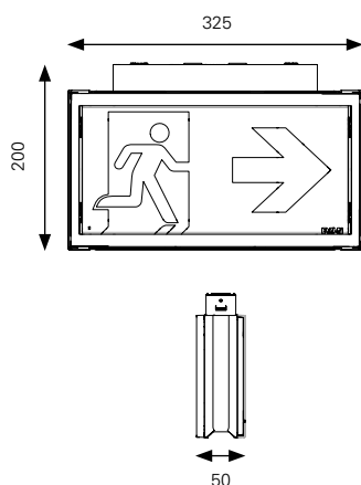
Massangaben (mm)
