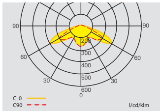
SL Atlantic LED O CGLine+ mit symmetrischer Optik
