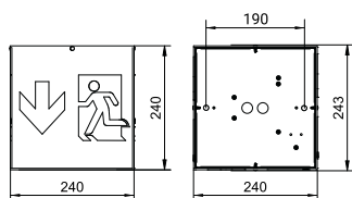
Technische Zeichnung
