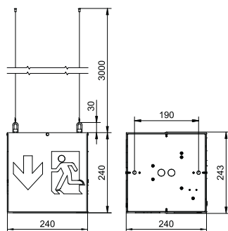
Technische Zeichnung
