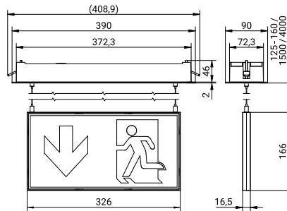
Technische Zeichnung
