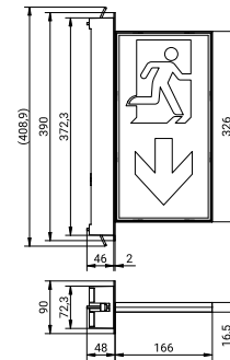
Technische Zeichnung
