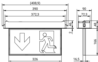
Technische Zeichnung
