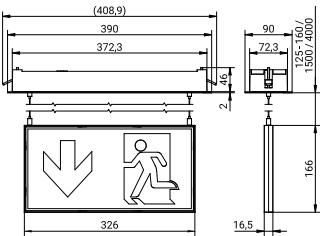
Technische Zeichnung
