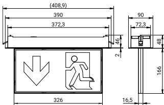
Technische Zeichnung
