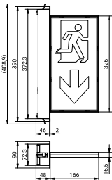
Technische Zeichnung
