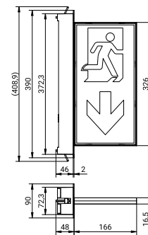
Technische Zeichnung
