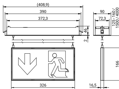
Technische Zeichnung
