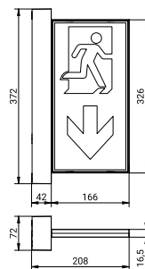
Technische Zeichnung
