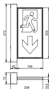
Technische Zeichnung
