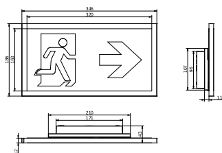
Technische Zeichnung
