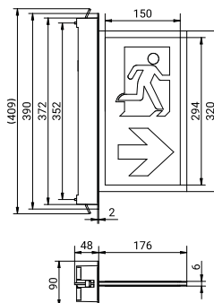
Technische Zeichnung
