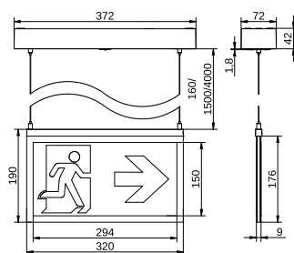
Technische Zeichnung
