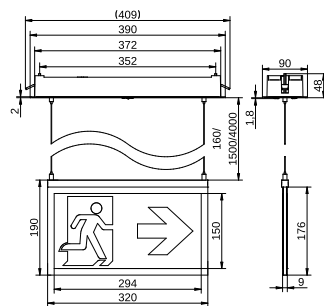
Technische Zeichnung
