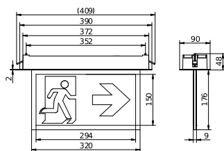
Technische Zeichnung
