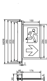
Technische Zeichnung
