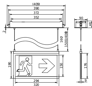
Technische Zeichnung
