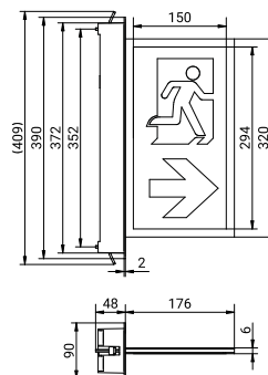
Technische Zeichnung
