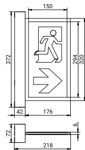
Technische Zeichnung
