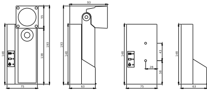
Technische Zeichnung
