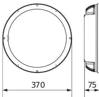
Technische Zeichnung
