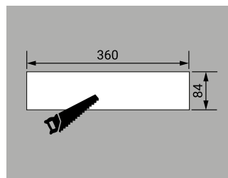
Ausschnitt
