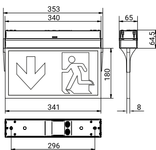
Technische Zeichnung
