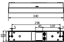
Technische Zeichnung
