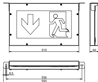
Technische Zeichnung
