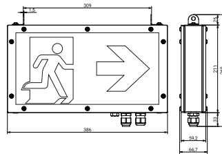
Set-Zeichnung für Ketten- oder Seilmontage
