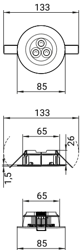
Technische Zeichnung
