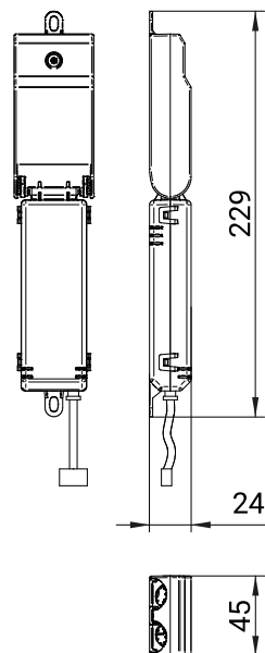
Technische Zeichnung
