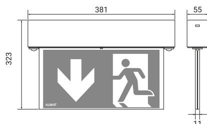
Technische Zeichnung
