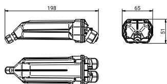
Technische Zeichnung
