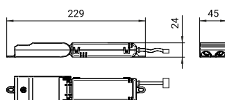
Technische Zeichnung
