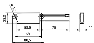
Technische Zeichnung
