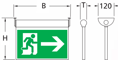
Deckenmontage, Pikto beidseitig
