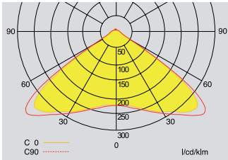
Lichtverteilungskurve i-P65+ L CGLine+
