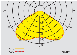
Lichtverteilungskurve SL 3583 1-8 h/D LED CGLine+
